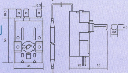
MTS 系列 尺寸圖
