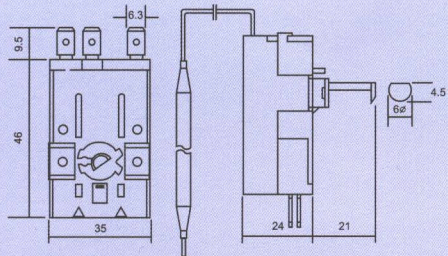
TS 系列 尺寸圖
